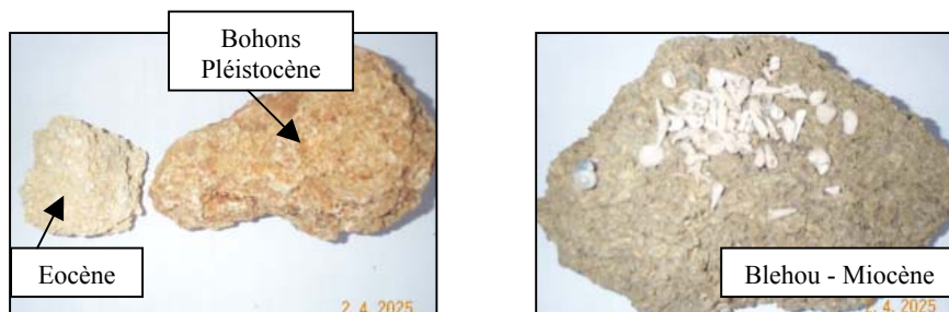
Les faluns aquifères de l'isthme du Cotentin
